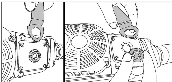
Рис. 4. Откручивание болта маслоналивной горловины
